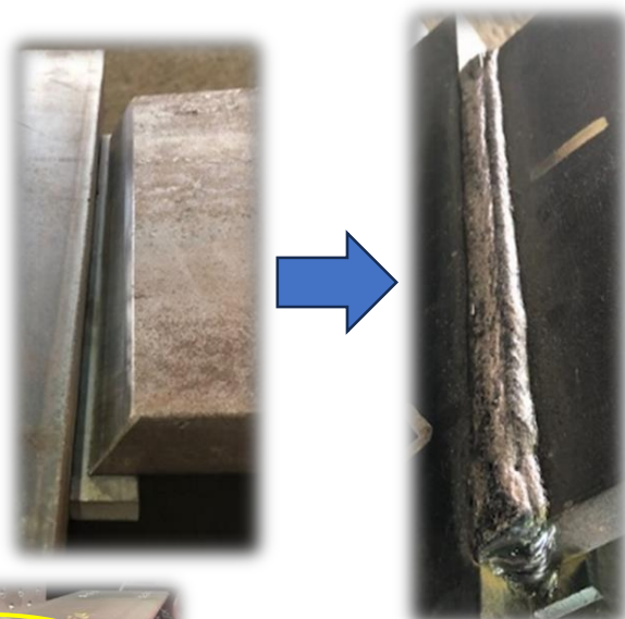
開先加工後の溶接部
